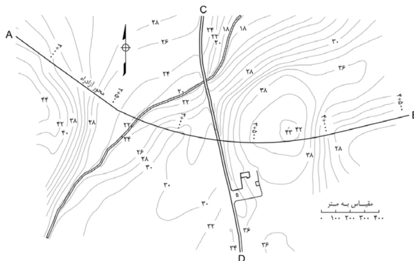
شکل ۹-۳۵- نقشه محل مورد نظر برای احداث تبادل
