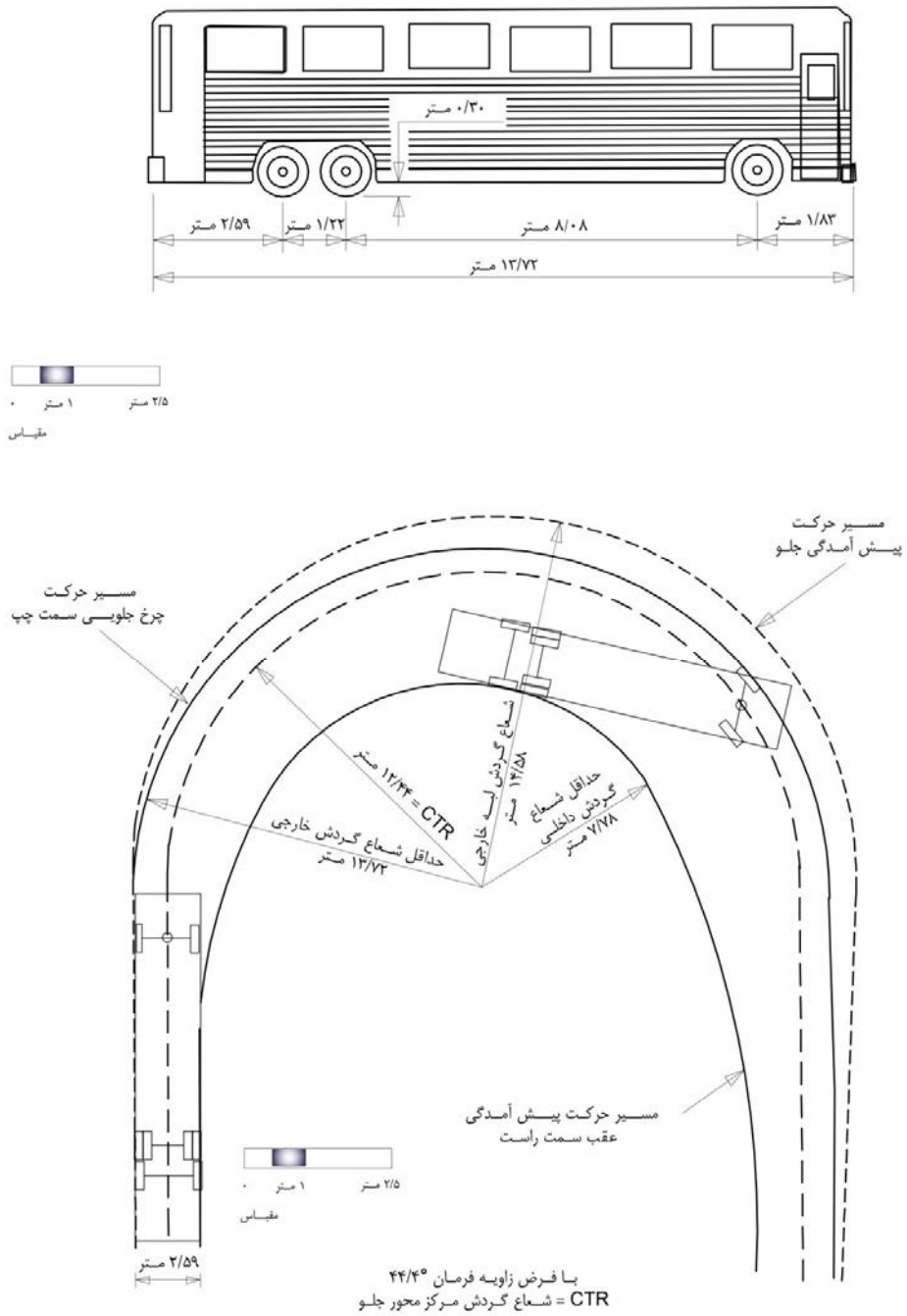
شکل ۳-۴ - مشخصات مسیر گردش خودروی طرح، اتوبوس نوع دوم
